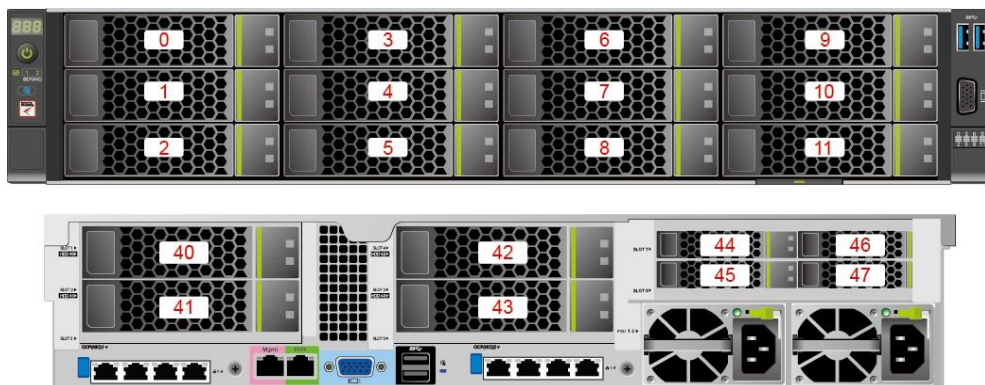
图 3-10 12x3.5 英寸硬盘 EXP 配置硬盘编号
