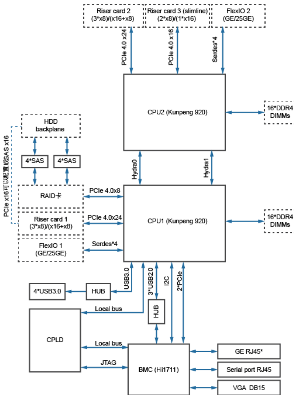
图 2-3 PR210K48逻辑结构
