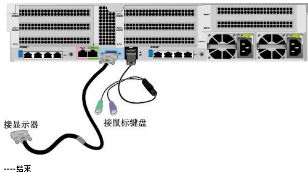
图 6-10 连接 USB 转 PS2 线缆和 VGA 接口
