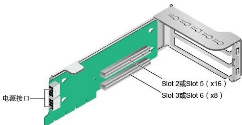
图 3-17 Riser 卡 2 ( 1x8+1x16 )
