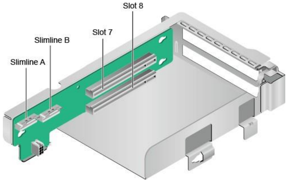
图 3-20 Riser 卡 6 ( 2x8 )
