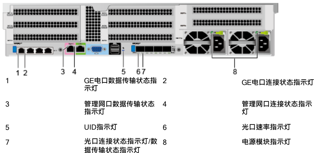
后面板指示灯
