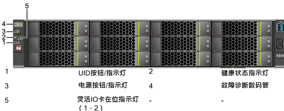
图 3-4 12x3.5 英寸硬盘配置前面板指示灯和按钮
