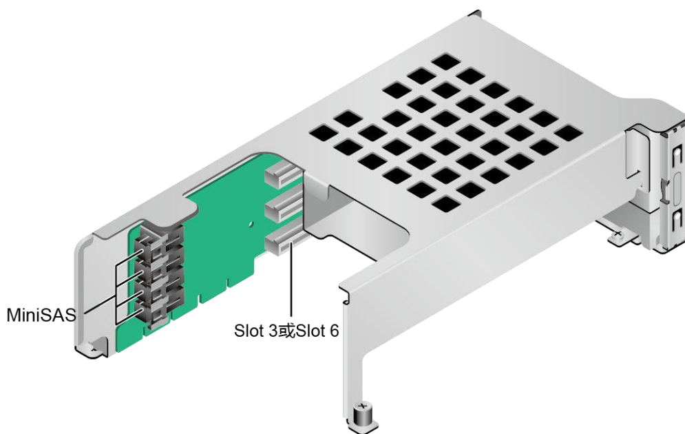
图 3-19 Riser 卡 5 ( SAS Riser )
