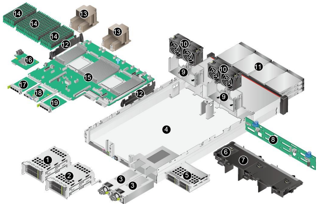
图 2-2 部件
