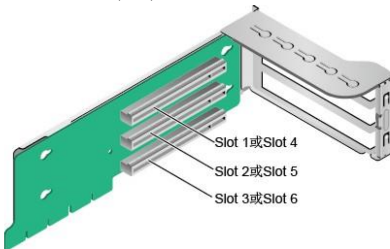
图 3-16 Riser 卡 1 ( 3x8 )
