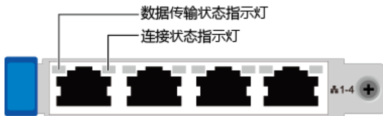
图 3-8 TM210 ( 4*GE 电口 )
