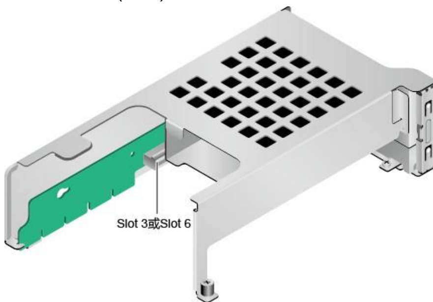
图 3-18 Riser 卡 4 ( 1x16 )
