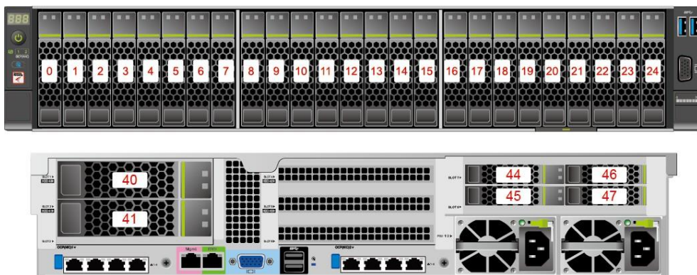
图 3-12 25x2.5 英寸硬盘 EXP 配置硬盘编号
