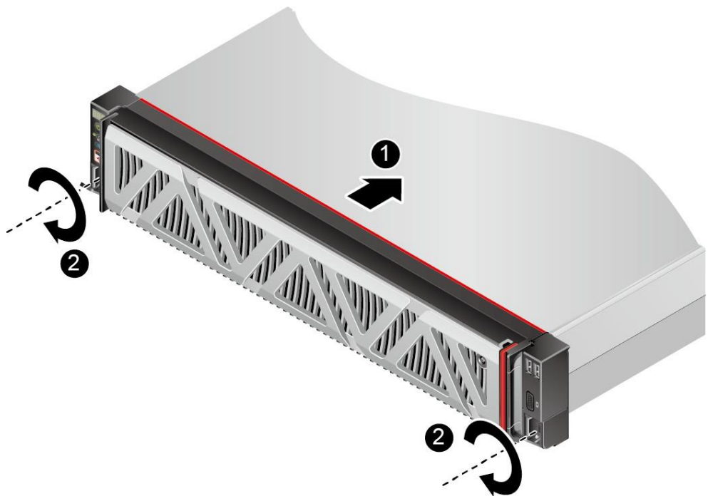
图 6-7 安装服务器
