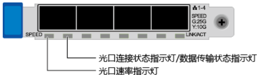
图 3-9 TM280 ( 4*25GE 光口 )
