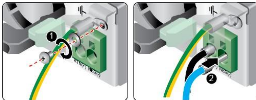
图 6-19 连接线缆
