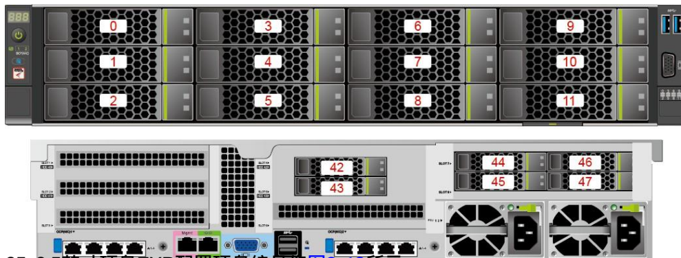
图 3-11 12x3.5 英寸硬盘直通配置
