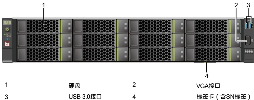
图 3-1 12x3.5 英寸硬盘配置前面板组件
