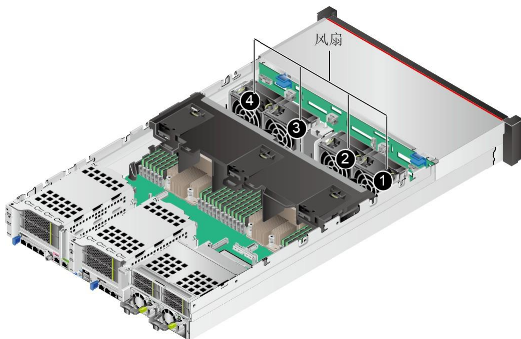
图 3-23 风扇位置图
