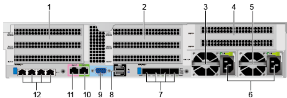
图 3-6 后面板组件
