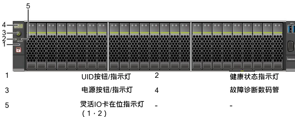
图 3-5 25x2.5 英寸硬盘配置前面板指示灯和按钮
