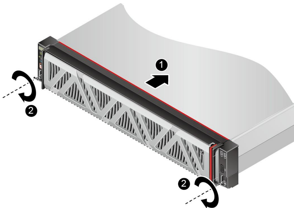
图 6-9 安装服务器
